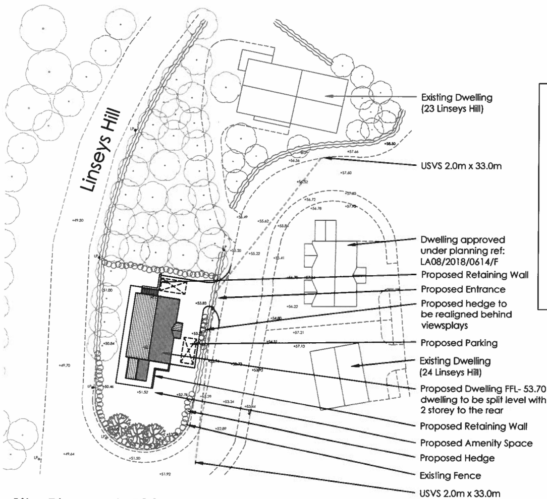
Site Plan 1:500
