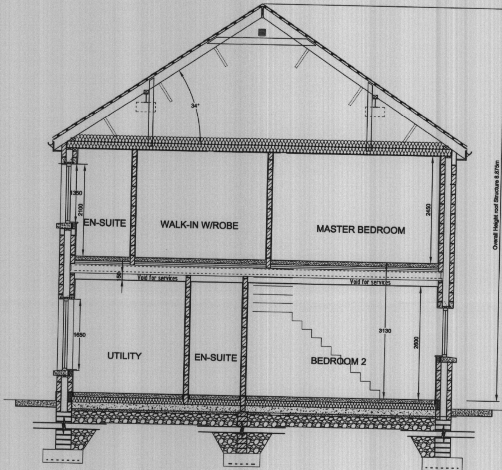
SECTION A-A
