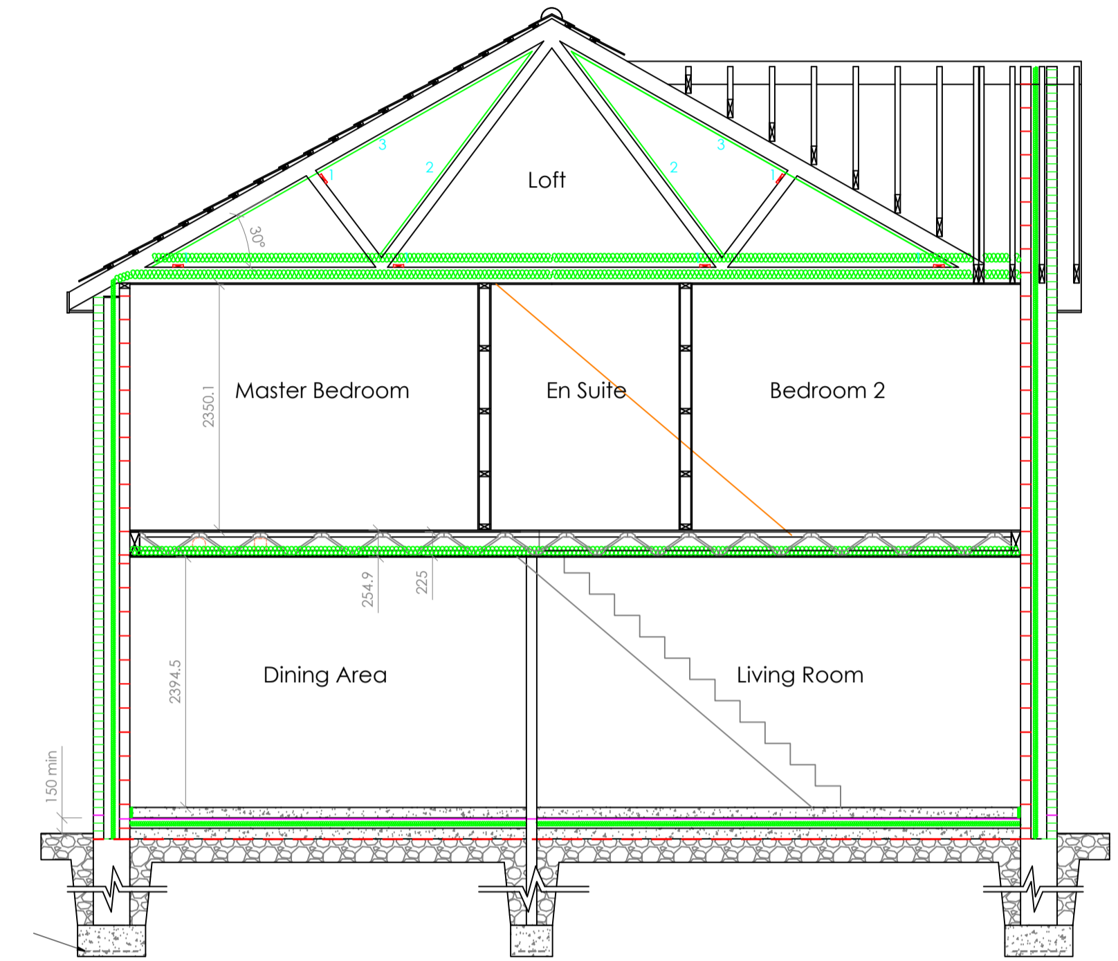
Section A-A
