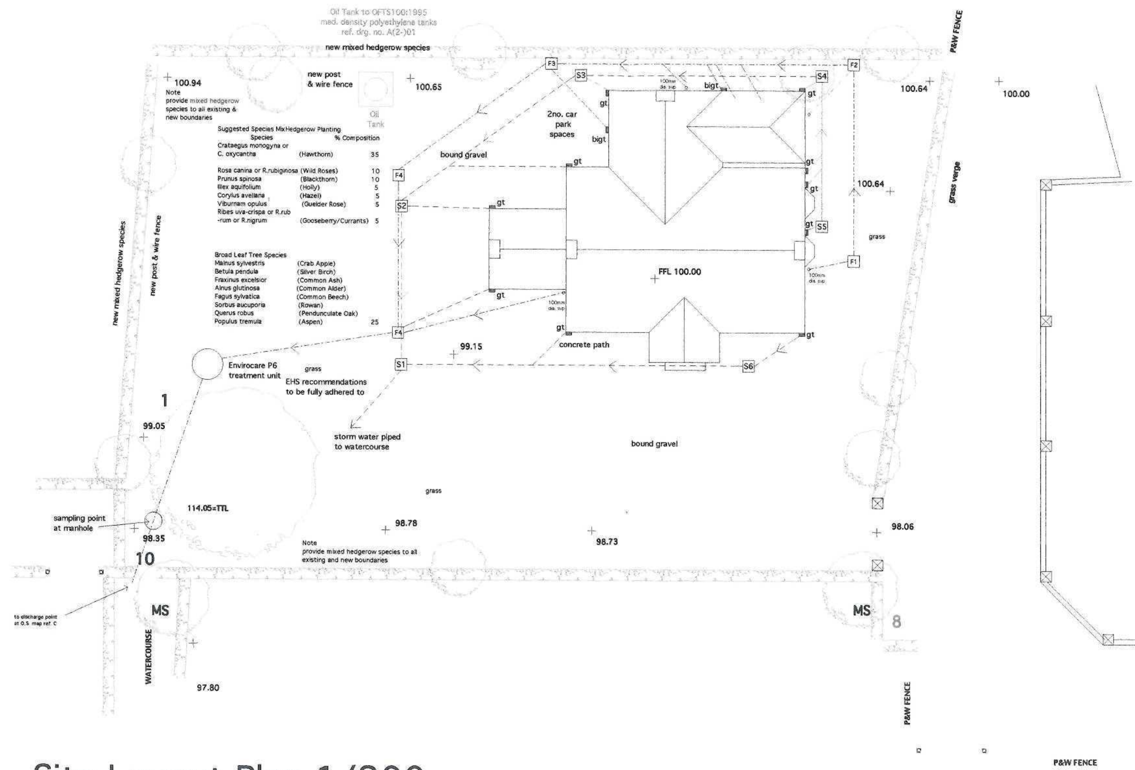
Site Layout Plan 1/200
